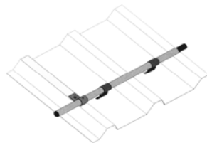
Einrohr-System
